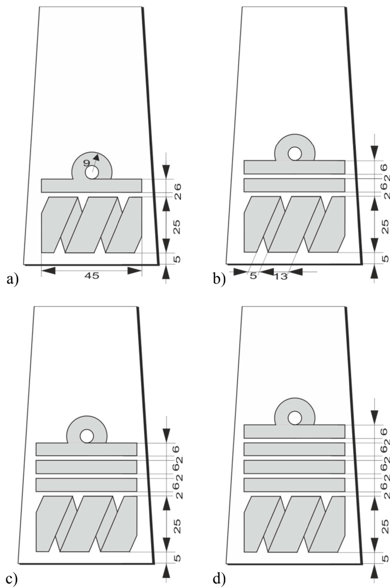
Rys. 14. Sposób rozmieszczania oznak stopni wojskowych na pochwecce
