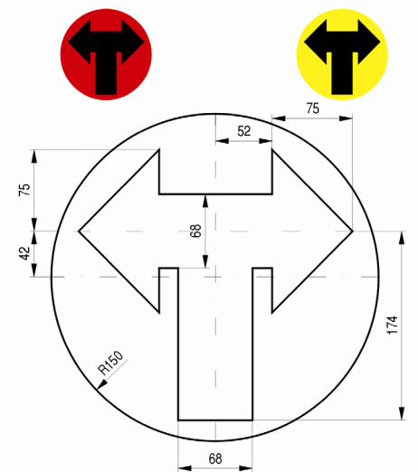
Rys. 10.8. Strzałki kierunku jazdy w prawo i w lewo dla sygnalu czerwonego i żółtego
