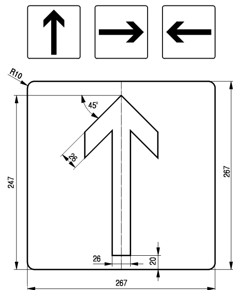
Rys. 10.24. Tabliczka kierunku jazdy na wprost albo w prawo lub w lewo dla tramwaju
