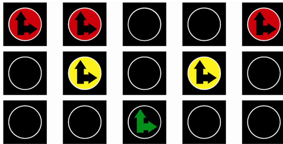
Rys. 4.2.6. Sygnalizatory kierunkowe S-3 i S-3a z sygnałami kierunkowymi na wprost i w prawo:
