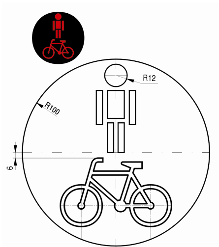
Rys. 10.23. Sylwetki pieszego i rowerzysty wspólnie w sygnale czerwonym; szablon pieszego według konstrukcji na rys. 10.20 należy zmniejszyć o 40%, a szablon roweru według konstrukcji na rys. 10.21 – o 30%
