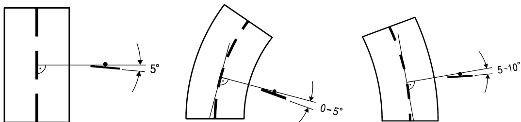
Rys. 1.5.5. Odchylenie poziome tarczy znaku:
