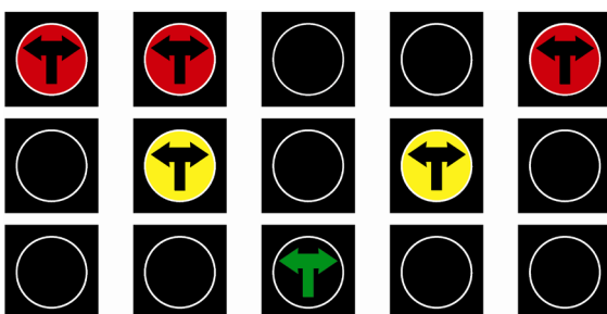
Rys. 4.2.7. Sygnalizatory kierunkowe S-3 i S-3a z sygnałami kierunkowymi w lewo i w prawo:
