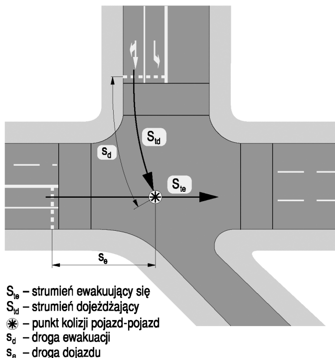
Rys. 8.3.1. Ilustracja pojęć związanych z obliczaniem czasu międzzielonego
